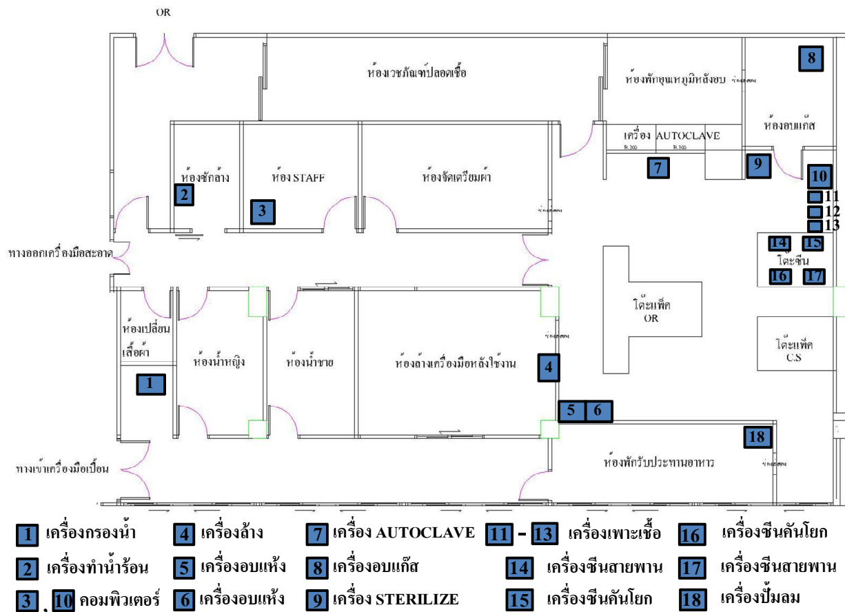
รูปที่ ข - 1 แสดงตำแหน่งเครื่องจักรและอุปกรณ์ไฟฟ้าที่อยู่ภายในแผนกจ่ายกลาง
