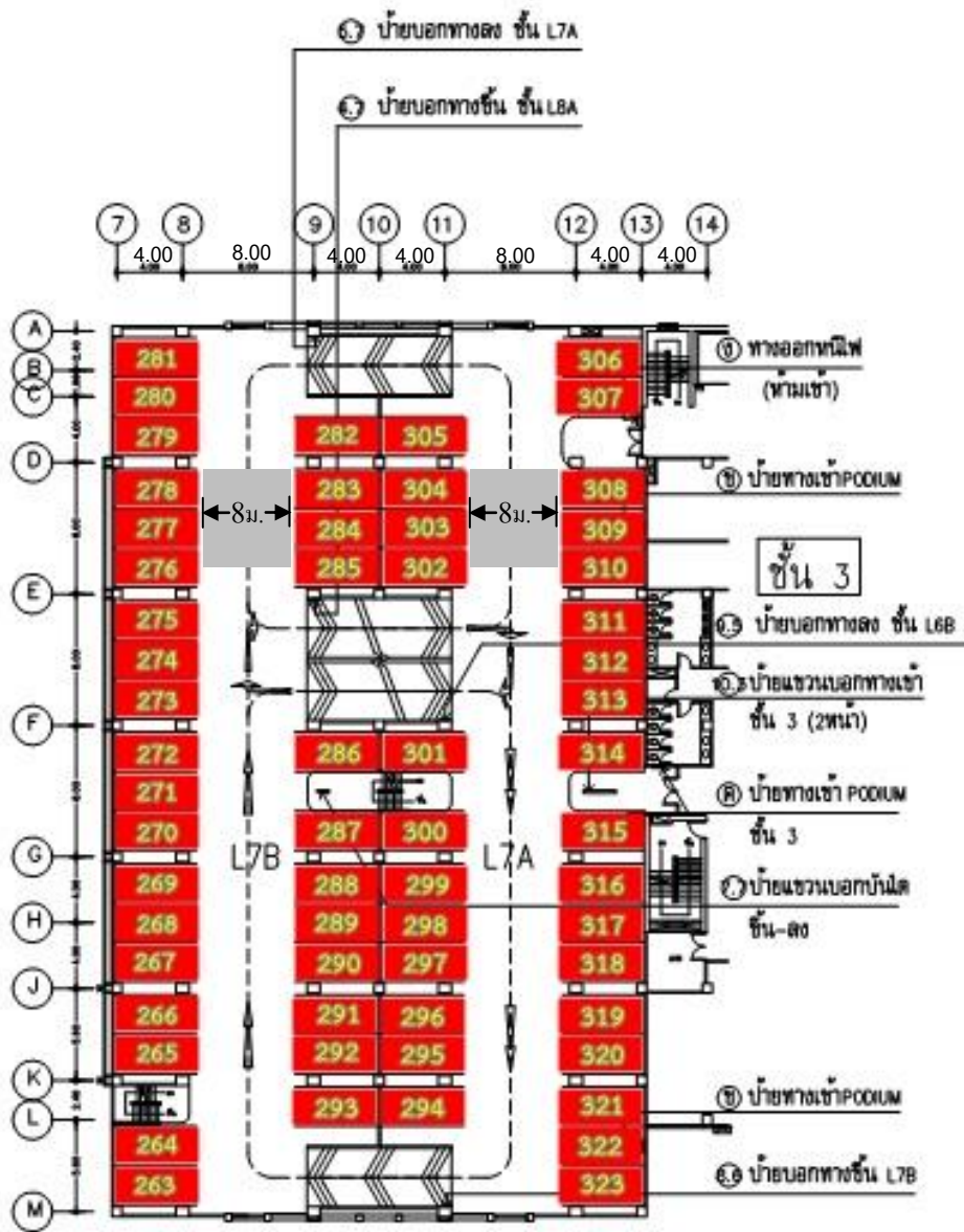
แปลนพื้นที่จอดรถชั้น L7A - L7B
