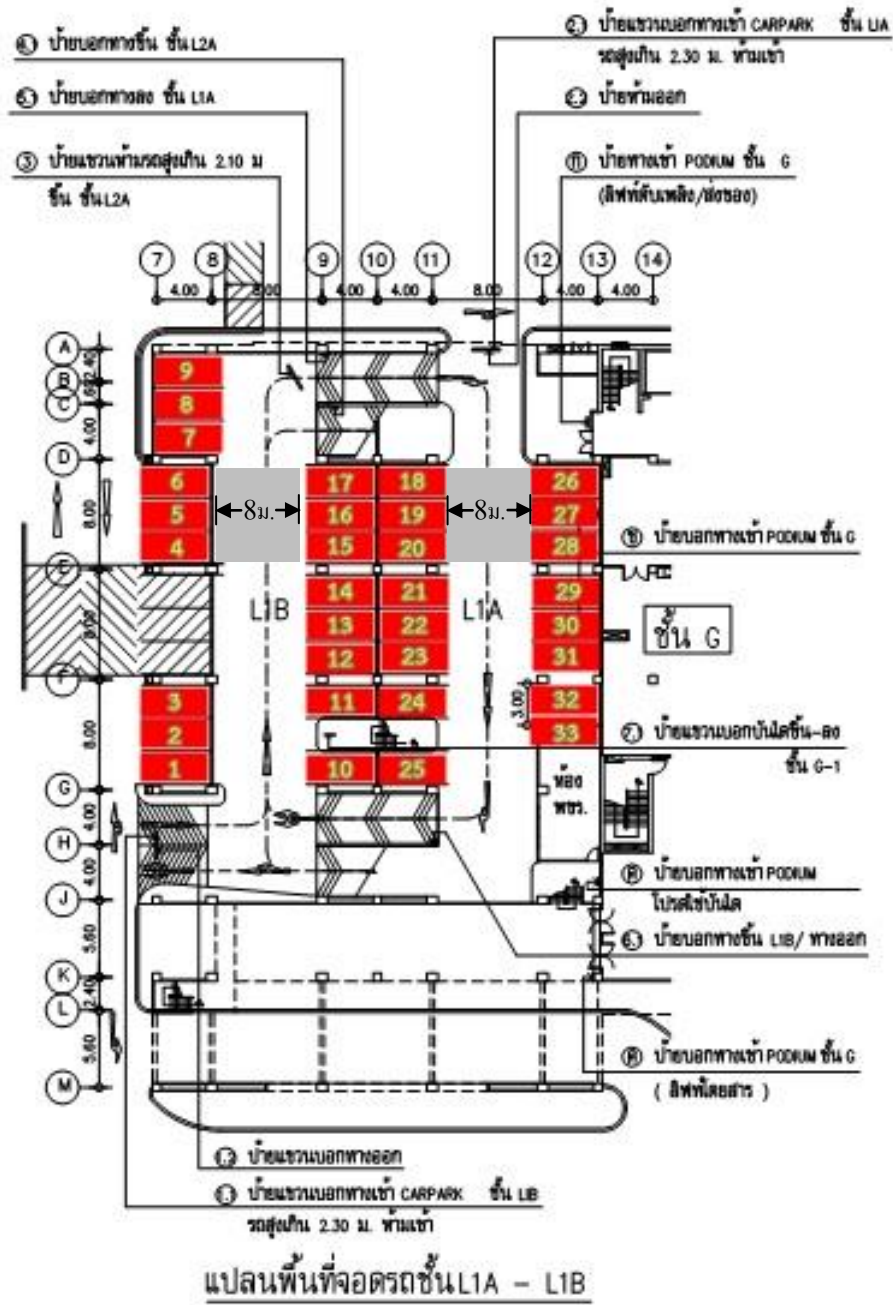
ภาพประกอบที่ 3 แปลนพื้นที่จอดรถชั้น L1A - L1B
