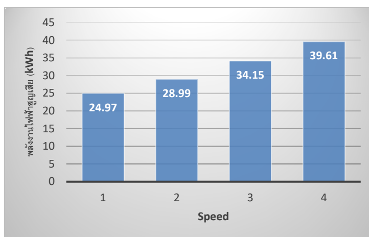
รูปที่ 7 การเปรียบเทียบการสูญเสียพลังงานไฟฟ้าจากการคำนวณการสูญเสียลมเย็นที่ทิ้งออกจากห้อง
