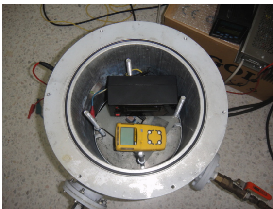
รูปที่ 4 การทดสอบการทำงานของเครื่องวัดที่ออกแบบเปรียบเทียบกับ GasAlert MicroClip
