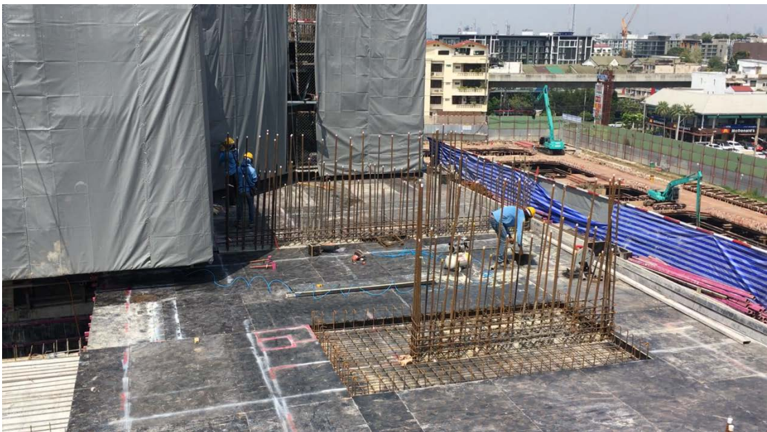
รูปที่ ค 2 ติดตั้งไม้แบบพื้น
