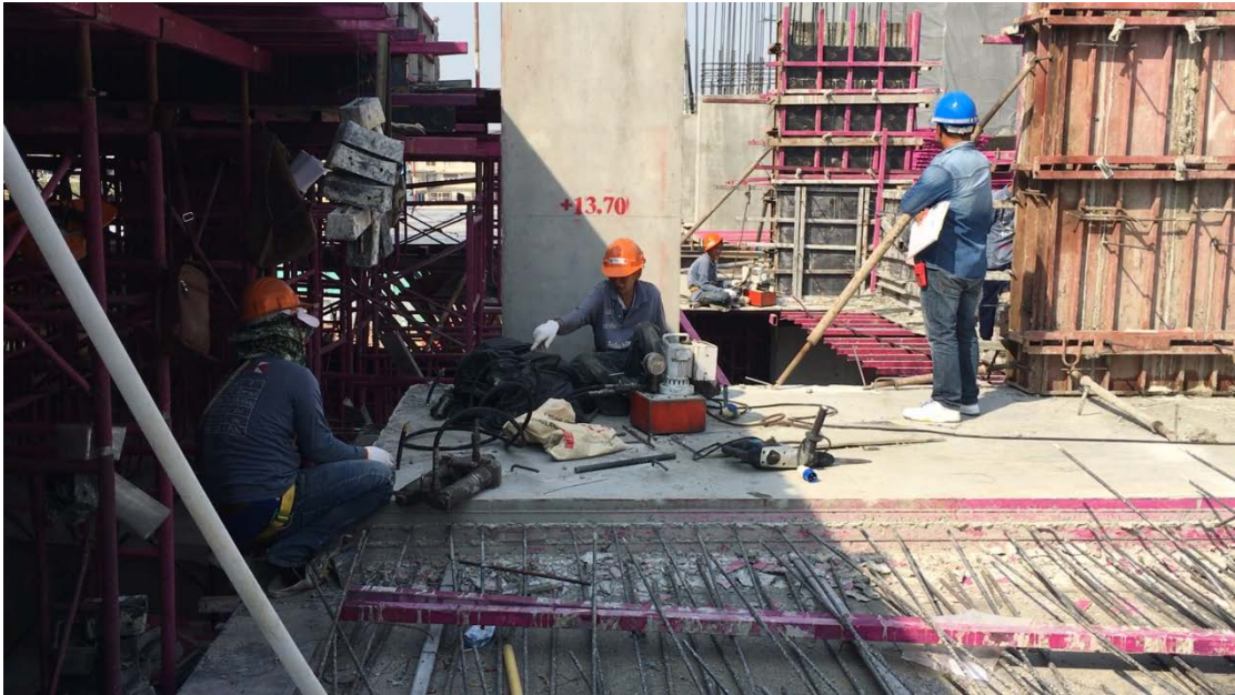
รูปที่ ค 7 ตั้งลวดสลิง
