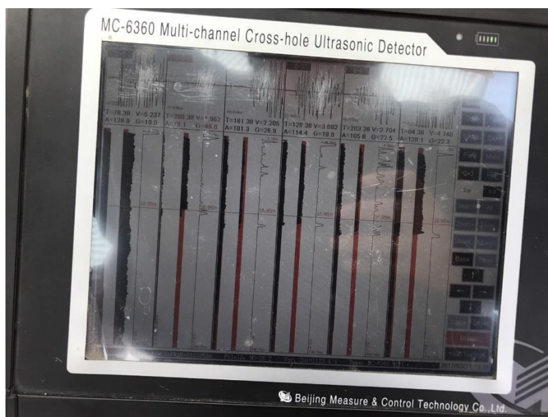
รูปที่ ก.8 ท่อSonic Logging เสียหาย
