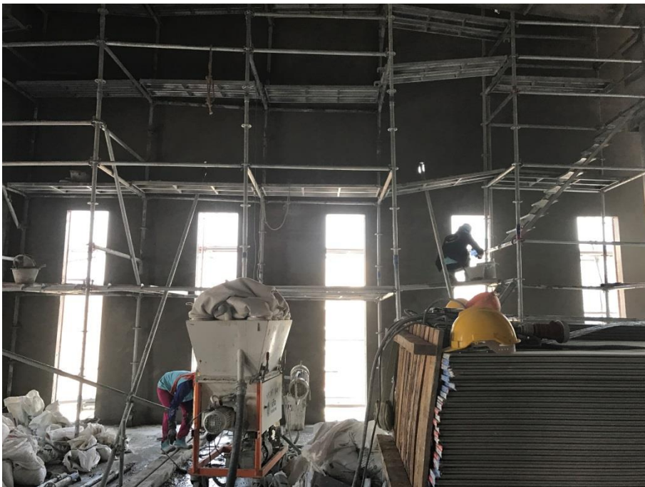
รูปที่ จ 14 แสดงกิจกรรมการขึ้นปูน/ปาดสามเหลี่ยม/ปั้นหน้าลงฟอง
