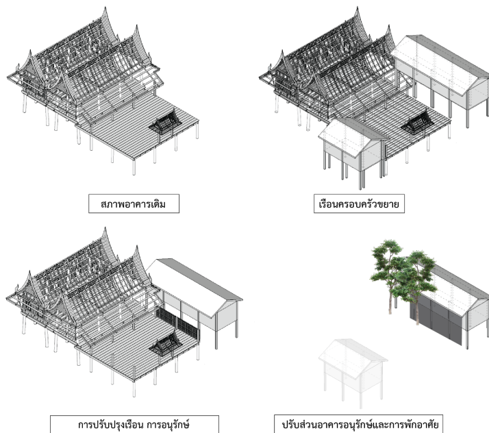
ภาพที่ 5 แสดงภาพจำลองเรือนด้วยโปรแกรมสร้างแบบ แนวทางการอนุรักษ์และบูรณะเรือนนายเซ่ง (จางเหยวียนเซ็ง) ที่มา: คณะผู้วิจัย
