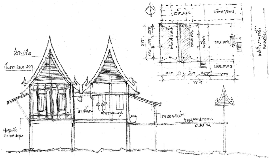
ภาพที่ 1 แสดงการสำรวจด้วยภาพวาด เรือนนายเซ่ง (จางเหยวียนเซ็ง)
