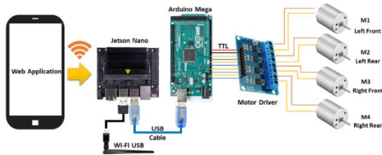
รูปที่ 2 ภาพแสดงการอินเตอร์เฟสของระบบเพื่อควบคุมมอเตอร์
